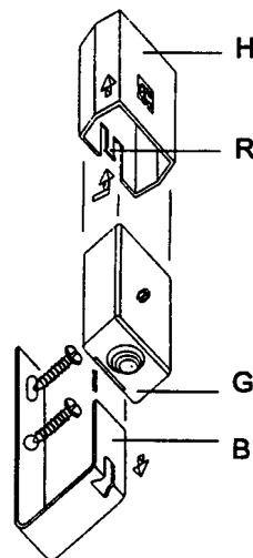
Рис. 2. Монтаж
