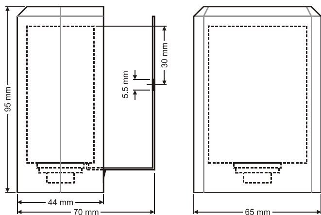
Рис. 1. Размеры (мм)
